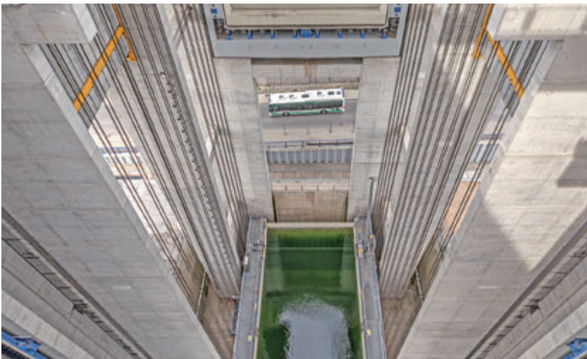
Blick in den Trog des neuen Schiffshebwerks
